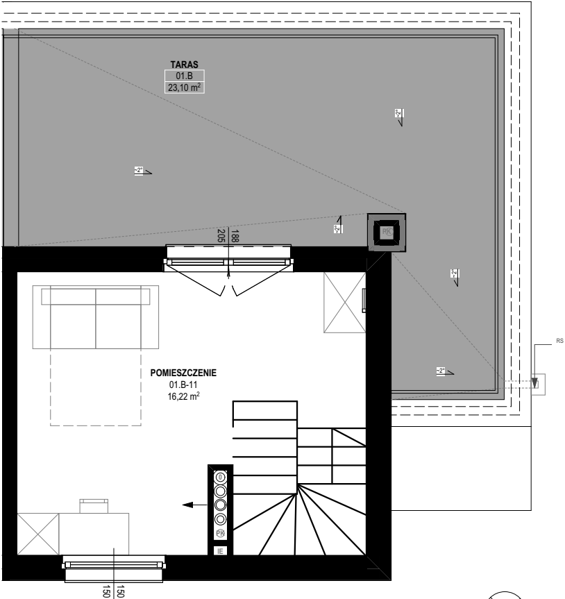
RZUT 2 PIĘTRA
