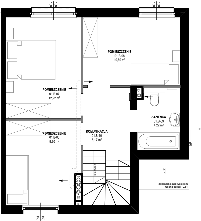
RZUT 1 PIĘTRA
