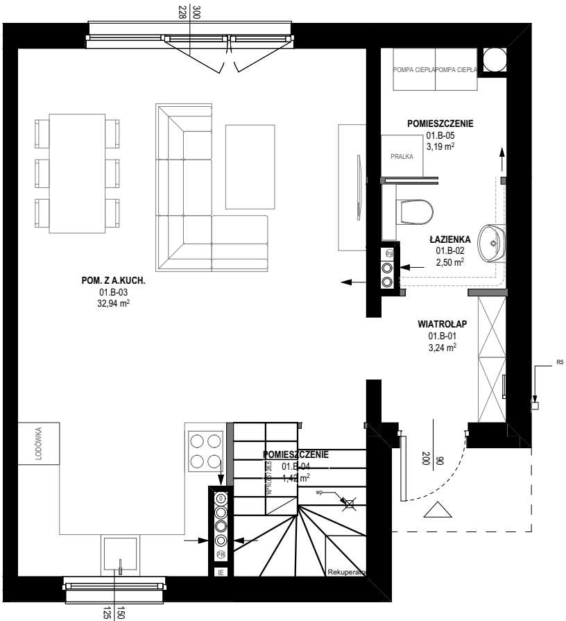
RZUT PARTERU
