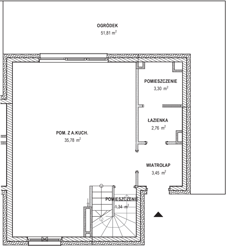
Kondygnacja: parter
