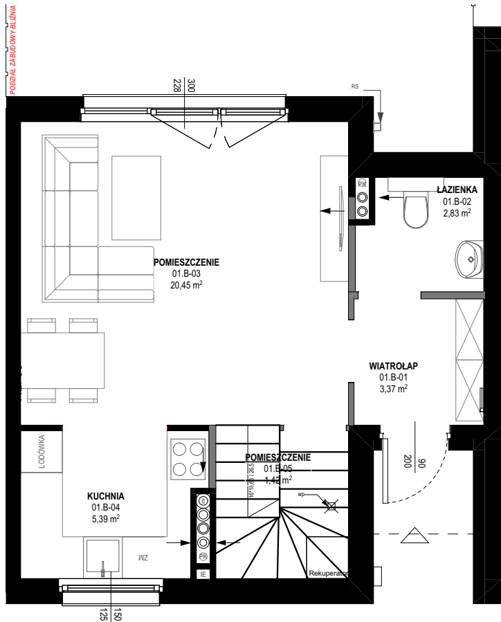
RZUT 1 PIĘTRA
