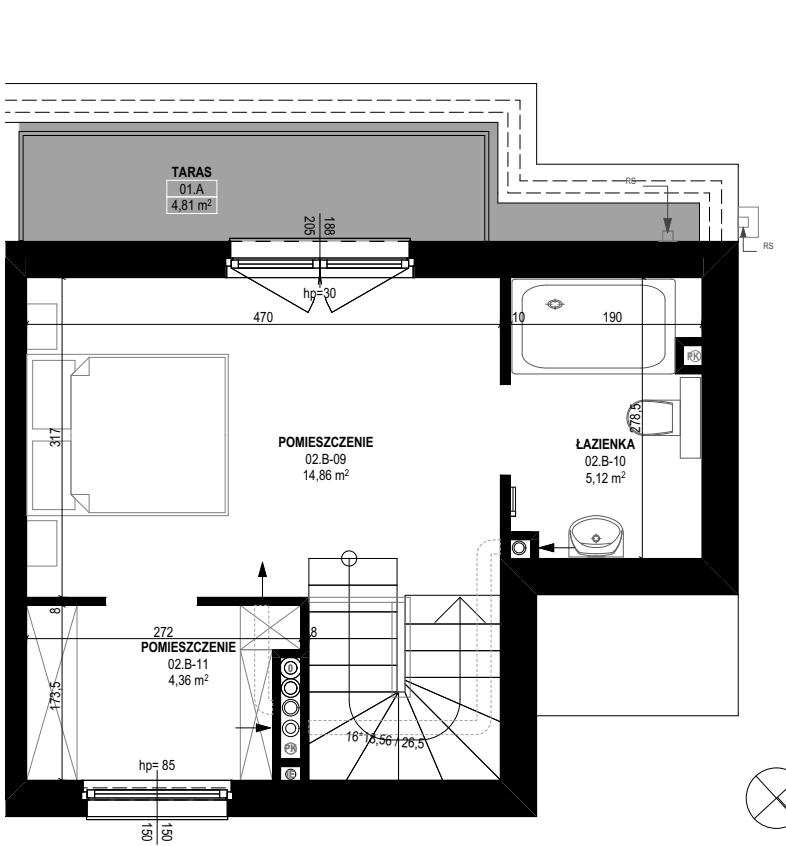
RZUT 2 PIĘTRA
