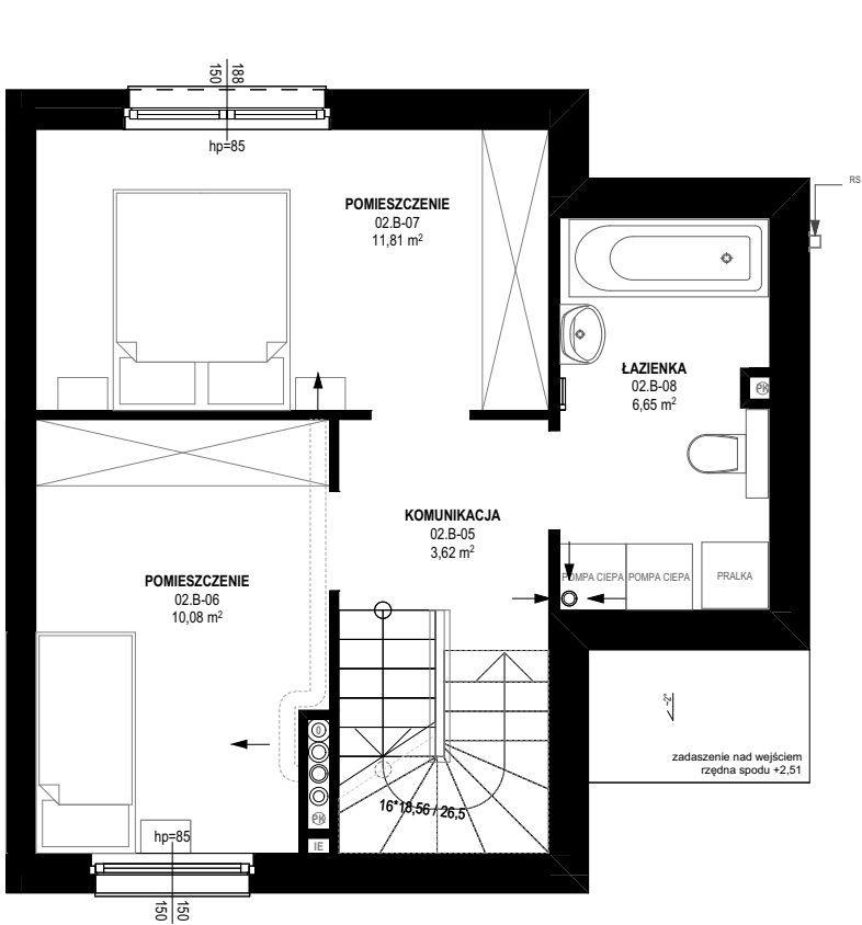
RZUT 2 PIĘTRA
