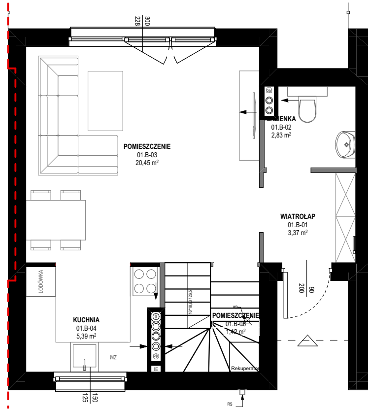
RZUT PARTERU
