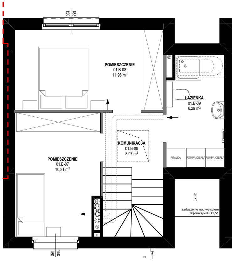
RZUT 1 PIĘTRA
