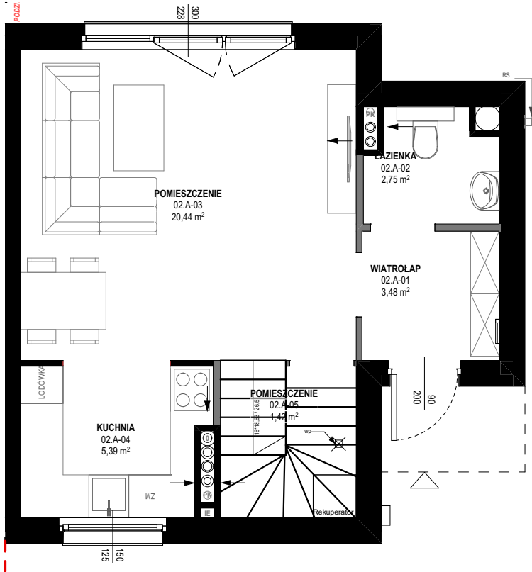
RZUT PARTERU
