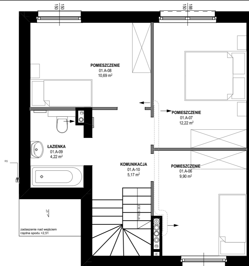
RZUT 1 PIĘTRA
