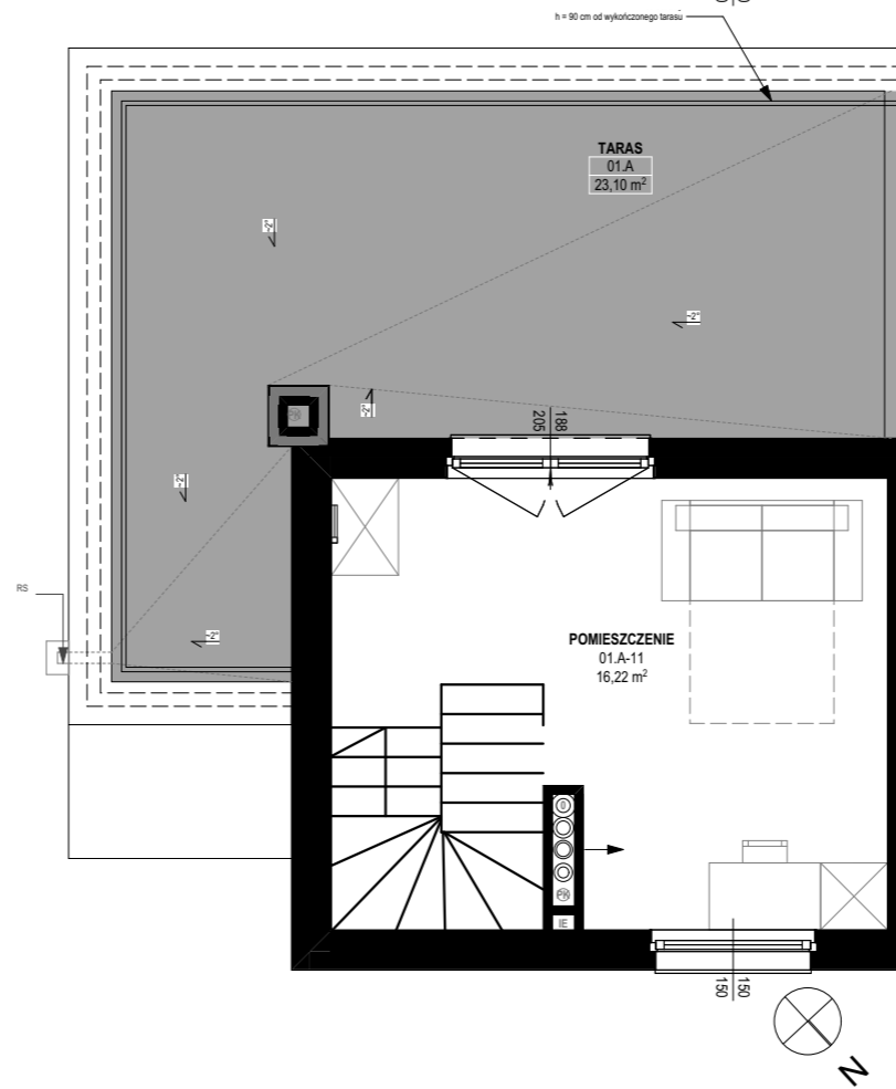
RZUT 2 PIĘTRA
